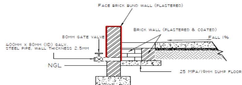
SUMP
