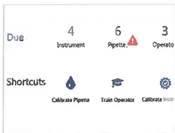
1. Identify pipette.
